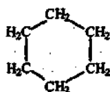
циклогексан
