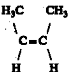
изс-бутен-2
