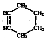
циклогексен
