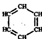
бензол
