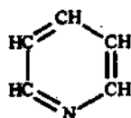
пиримидин
