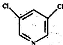
3,5-дихлорпиридин
