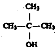
метилпропанол-2 (третичный)
